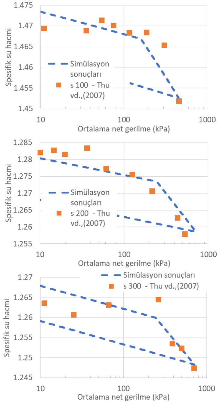
Şekil 7. Spesifik su hacminin net gerilmeye göre değişimlerinin üç emme değerinde modellenmesi
