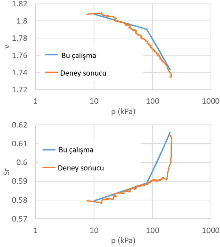
Şekil 10. Elazığ siltiyle 40 kPa sabit emmede yapılan izotropik sıkıştırma deneyi ve bünye modeli sonuçları
