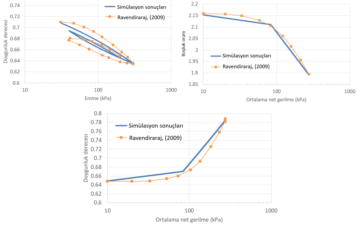
Şekil 8. İzotropik sıkışma ve karşı gelen doygunluk derecesi davranışlarının Ravendiraraj, (2009) deneyleri ile simülasyonu
