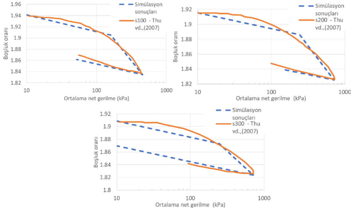
Şekil 6. Model sonuçları ile Thu vd. (2007) deneylerinin üç farklı emmede (s, kPa) karşılaştırılması
